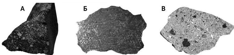
Рис. 2.2. Спилы метеоритов:
