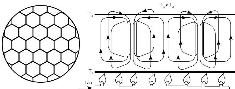
Рис. 5.4. Ячейки Бенара
