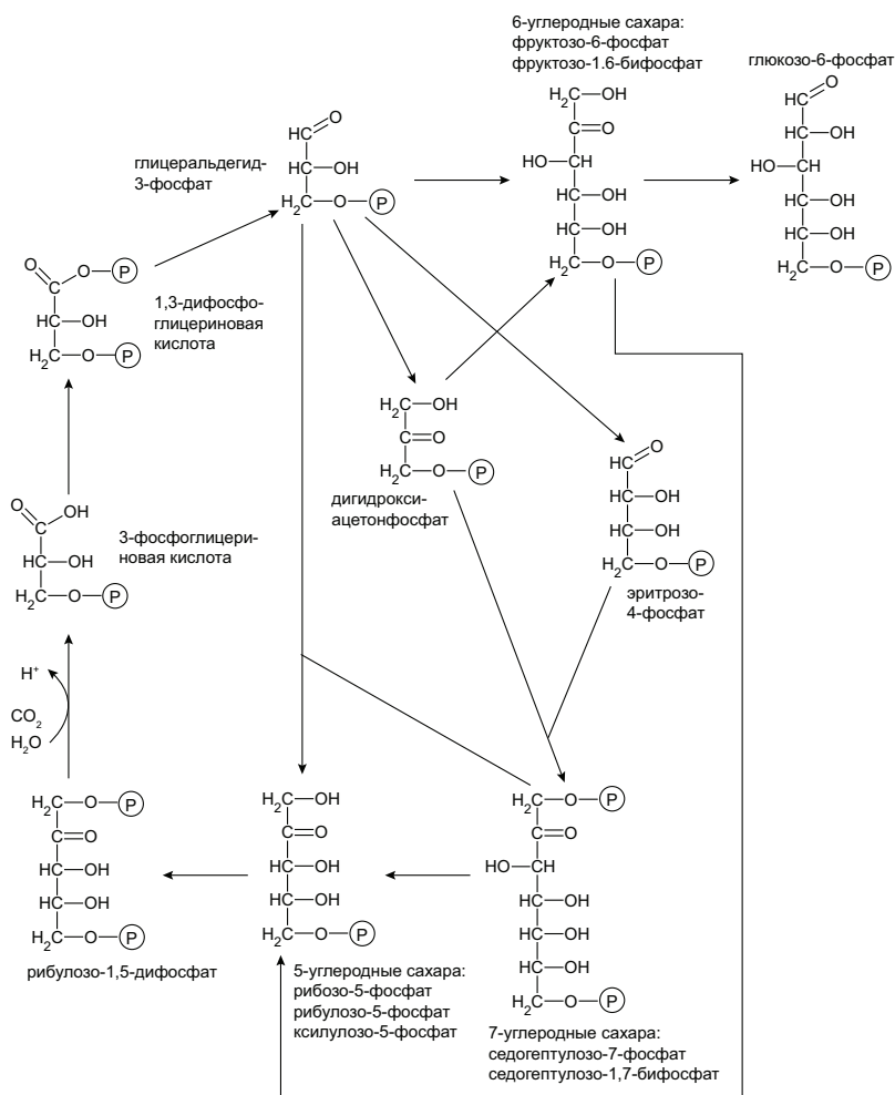
Рис. 11.2. Упрощенная схема цикла Кальвина
