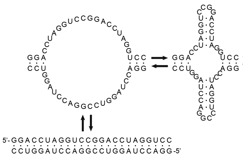
Рис. 9.6. Альтернативные способы укладки РНК, содержащей палиндромные повторы
