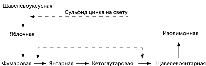
Рис. 11.6. Реакции восстановительного цикла Кребса на кристаллах ZnS
