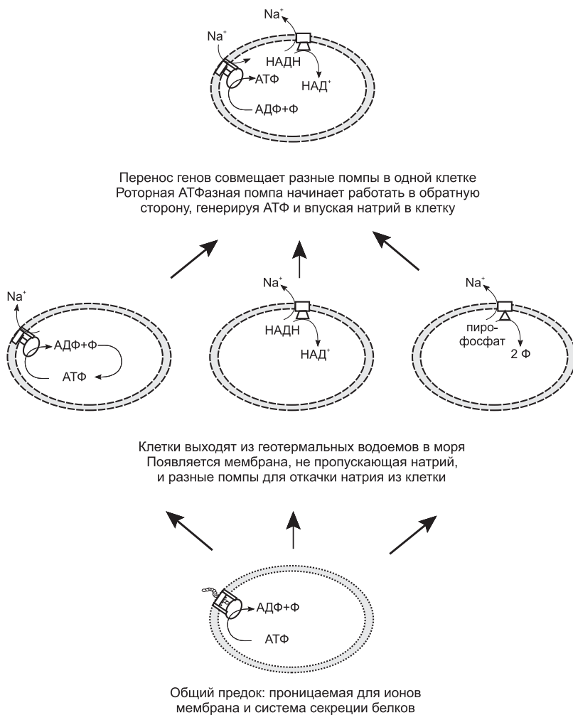
Рис. 15.12. Схема эволюции мембран и мембранной энергетики.
