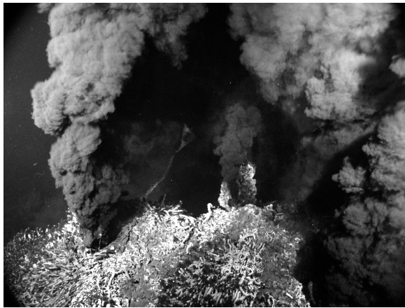
Рис. 6.3. Схема и фотография «черных курильщиков»
